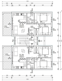
TLOCRT KROVNÍH PLOHA M 1:100
