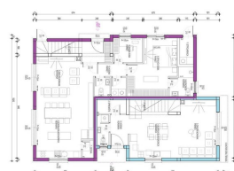
TLOCRT PRIZEMLJA
