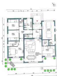
TLOCRT PRIZEMLIA
