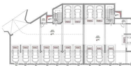
Půdorys suterénu
