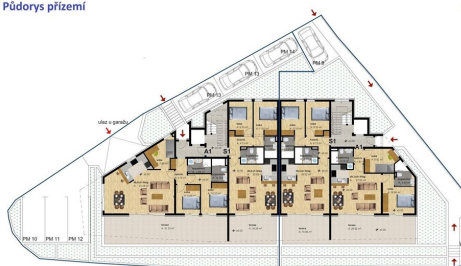
Půdorys přízemí
